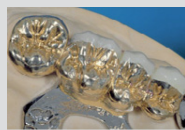
20 und 21 Der Schwenkriegel integriert sich hervorragend in das Gesamtkonstrukt. Die Fingernagelraste wurde approximal platziert, wo sie keine Störungen und Irritationen verursacht.
