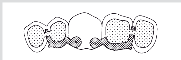
18 In der Kronenwand integrierte Schwenkhebel mit interproximaler Arretierung.
