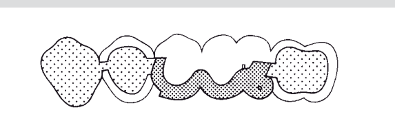
19 Die schematische Darstellung der Doppelverriegelung zeigt die Lage des Schwenkhebels zu den Stegstummeln und dem Anschlag.
